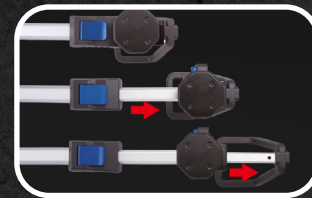
SUPORTE COM 3 AJUSTES DE COMPRIMENTO
