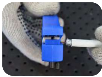
Desencapa cabos coaxiais sem danificar a manta
